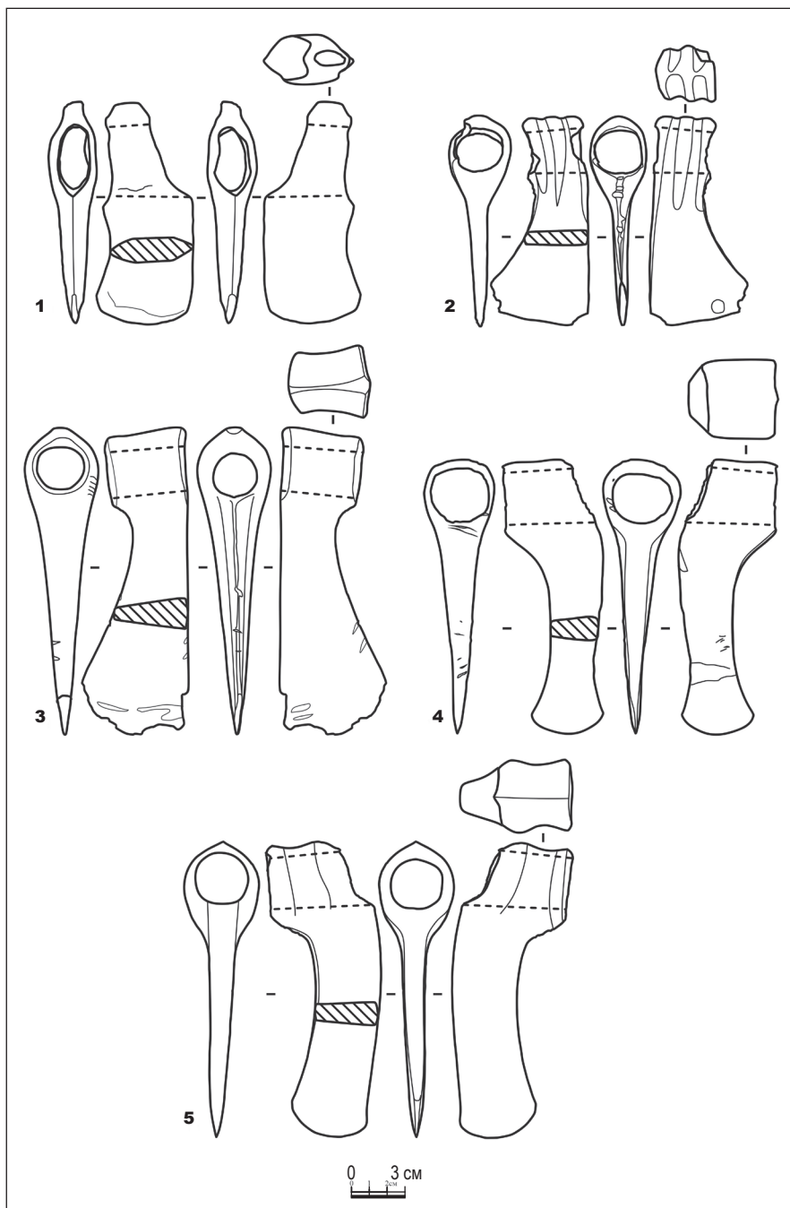
Рис. 1. Топоры из Абхазского государственного музея, рисунки: 1 – Кула- нурхва; 2 – Азанта; 3 – Члоу; 4–5 – Лечкоп.
