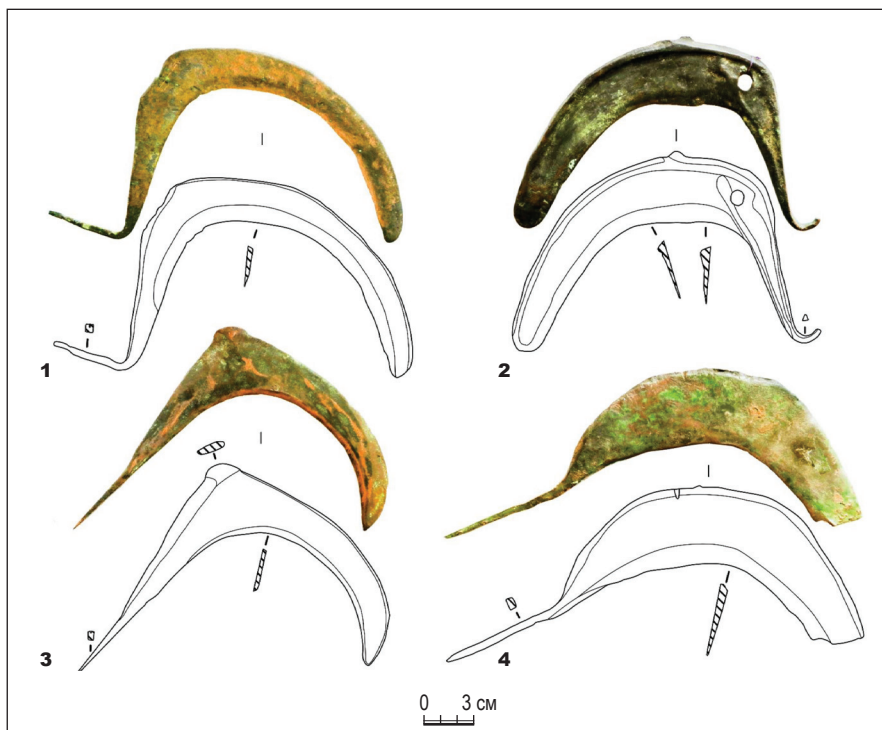
Рис. 1. Серпы из музея историко-культурного наследия CAO РАН и Нижнего Архыза, фото и рисунки.
